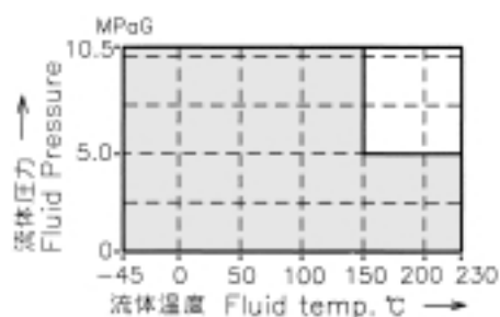
Fig. 2-1 LOW TORQUE TYPE : TFE CARBON FIBER
