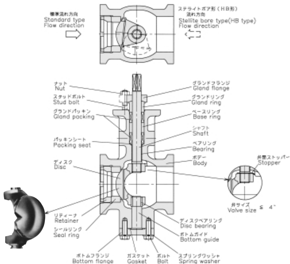
Fig. 4-1 M CLASS BODY STANDARD TYPE : JIS10K, 20K, 30K / ANSI (JPI) CLASS 150, 300
